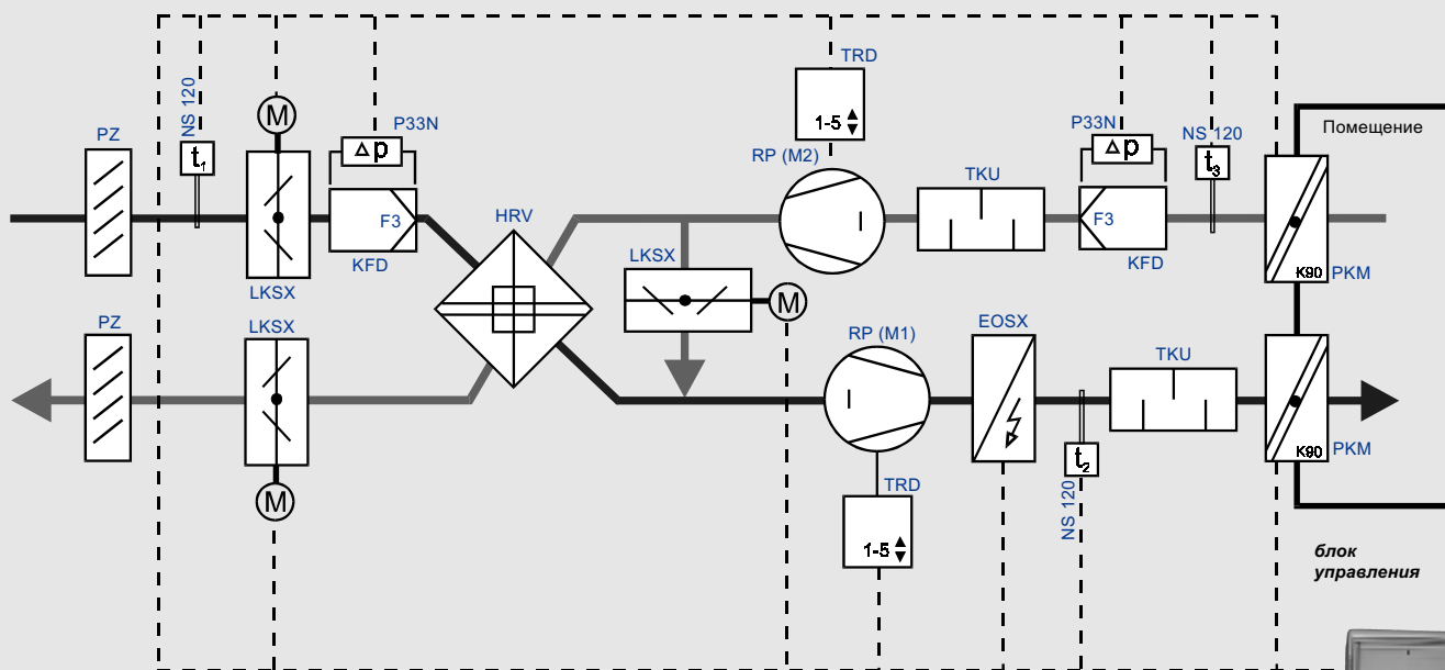
Рис. 14 – рекуператор без байпаса
