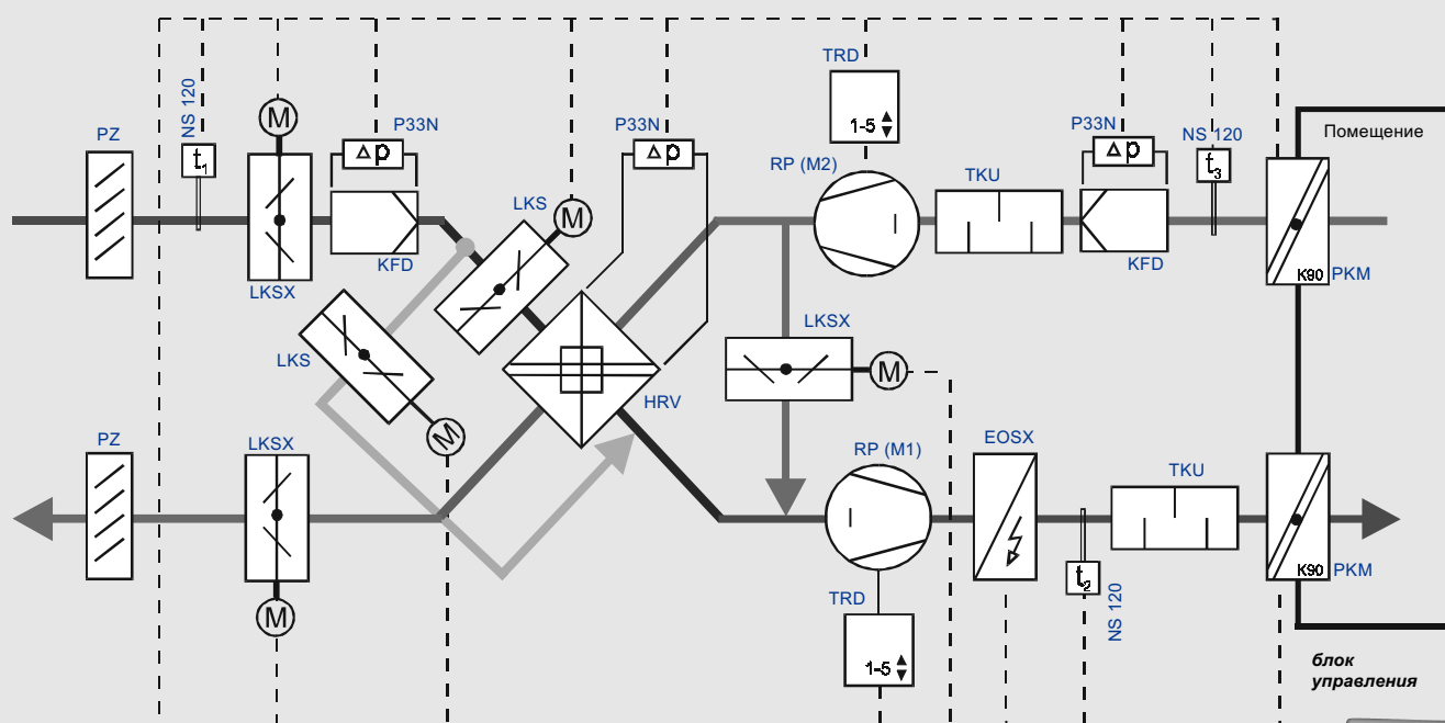
Рис. 15 – рекуператор с байпасом
