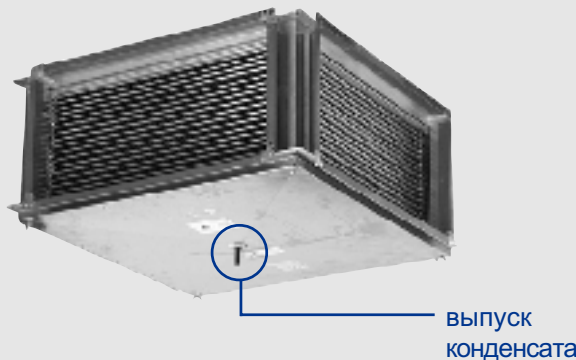
Рис. 9 – PVC выпуск
